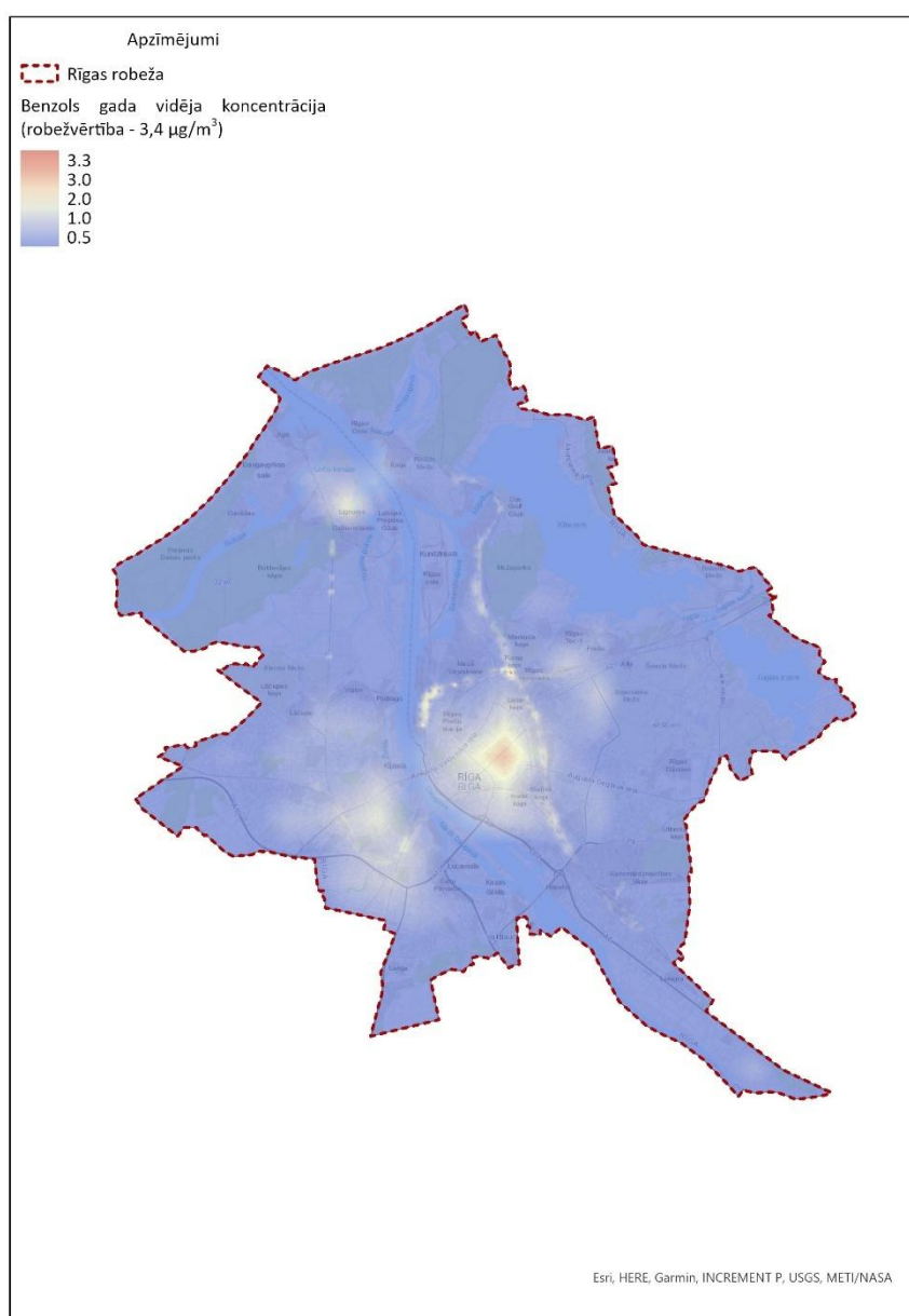
5.3.1. attēls. Benzola piesārņojuma izkliede – gada vidējās koncentrācijas 2023. gadā
