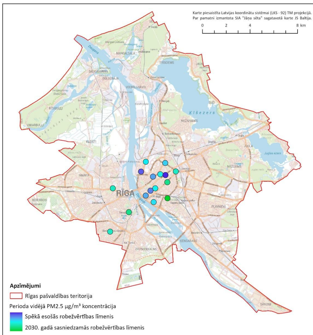
3.2.2. attēls. Urban Relief projekta ietvaros veiktā daļiņu PM_{2,5} indikatīvā (sensoru) monitoringa rezultāti, 2024. gada marts – 2025. gada marts (Avots: PurpleAir 36 )
