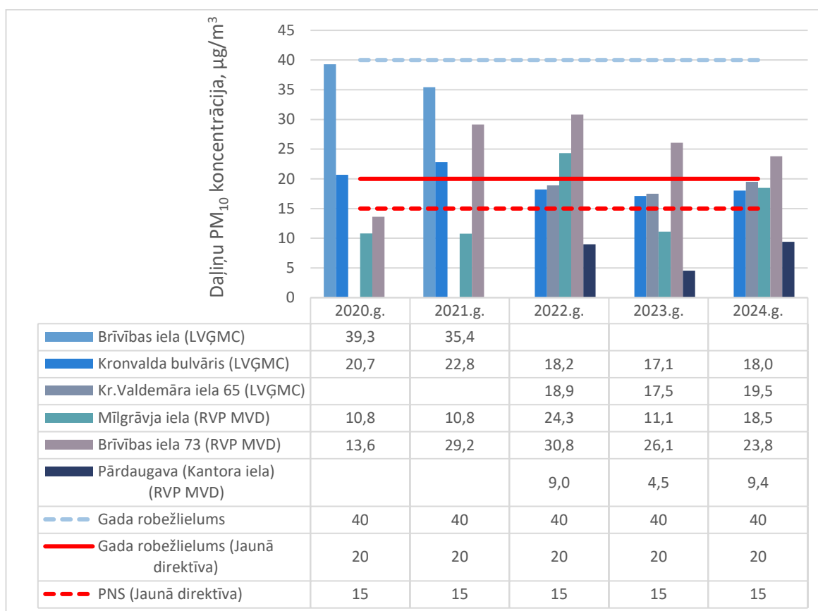
3.1.6. attēls. Gada vidējās daļiņu PM 10 koncentrācijas Rīgā 2020.-2024. gadā (avots: LVĢMC, RVP MVD)
