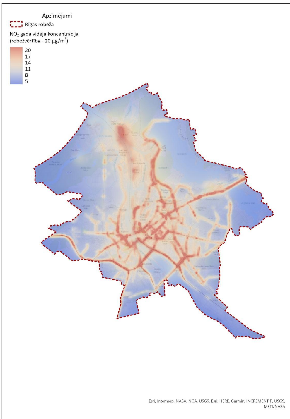
8.1. attēls. Aprēķinātā slāpekļa dioksīda gada vidējā koncentrācija 2030. gadā, atbilstība robežlielumam atbilstoši Direktīvai 2024/2881 jānodrošina līdz 01.01.2030. (scenārijs ar pasākumiem)
