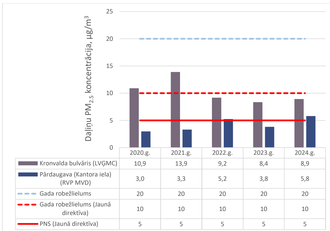
3.1.7. attēls. Gada vidējās daiļņu PM 2,5 koncentrācijas Rīgā 2020.-2024. gadā (avots: LVĢMC, MVD)
