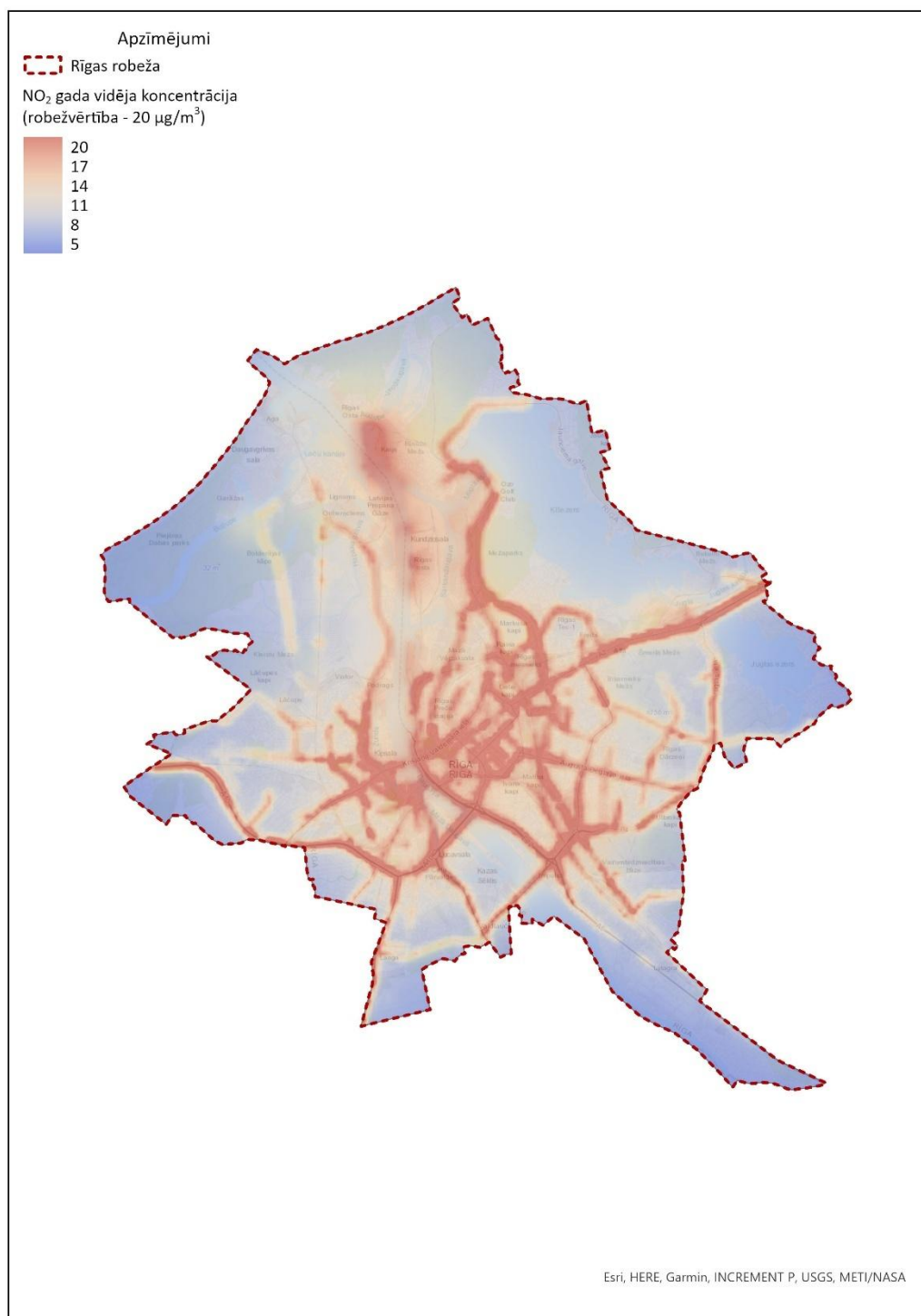
6.2.1. attēls. Aprēķinātā slāpekļa dioksīda gada vidējā koncentrācija 2030. gadā (bāzes scenārijs)
