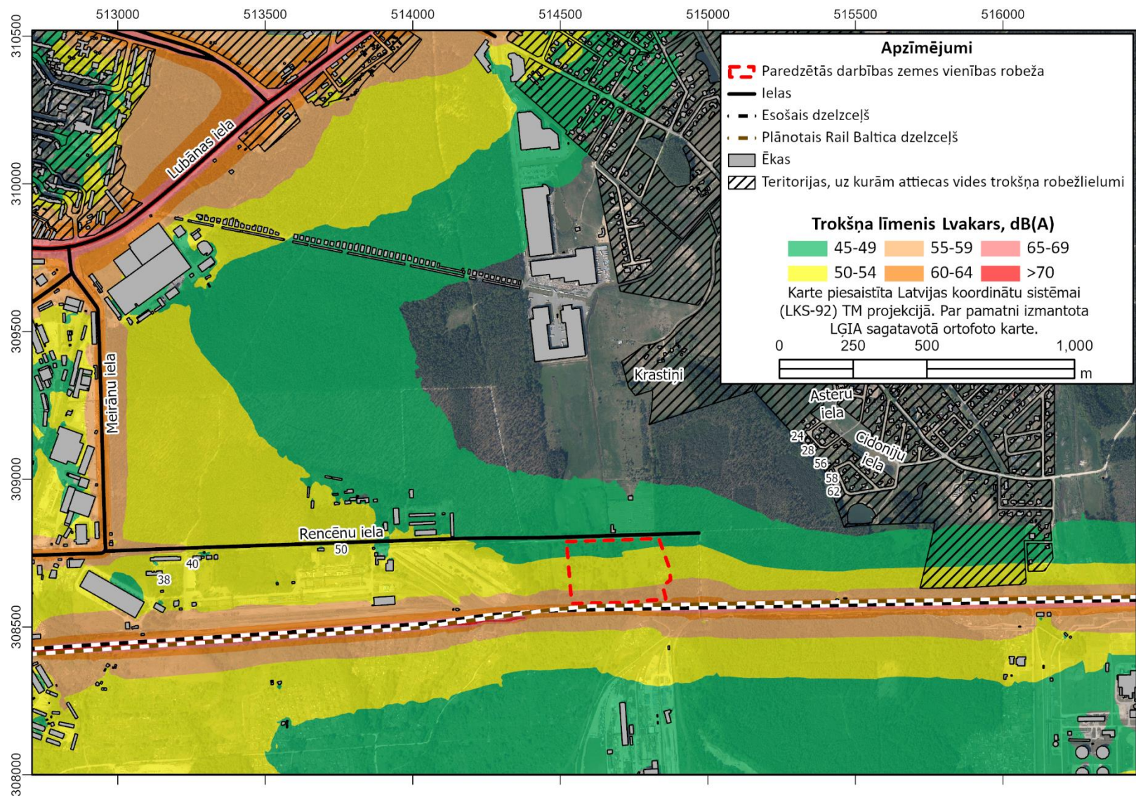
2. attēls. Aprēķinātais fona trokšņa līmenis trokšņa rādītājam L_{vakars}
