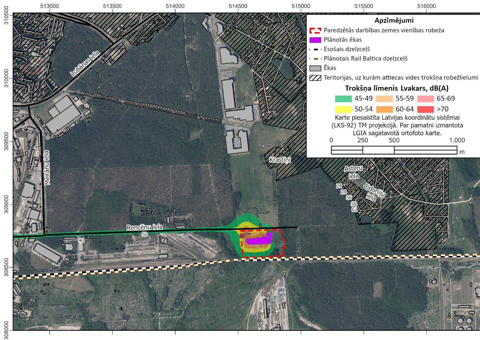
5. attēls. Plānotās darbības radītais trokšņa līmenis trokšņa rādītājam L_{vakars}
