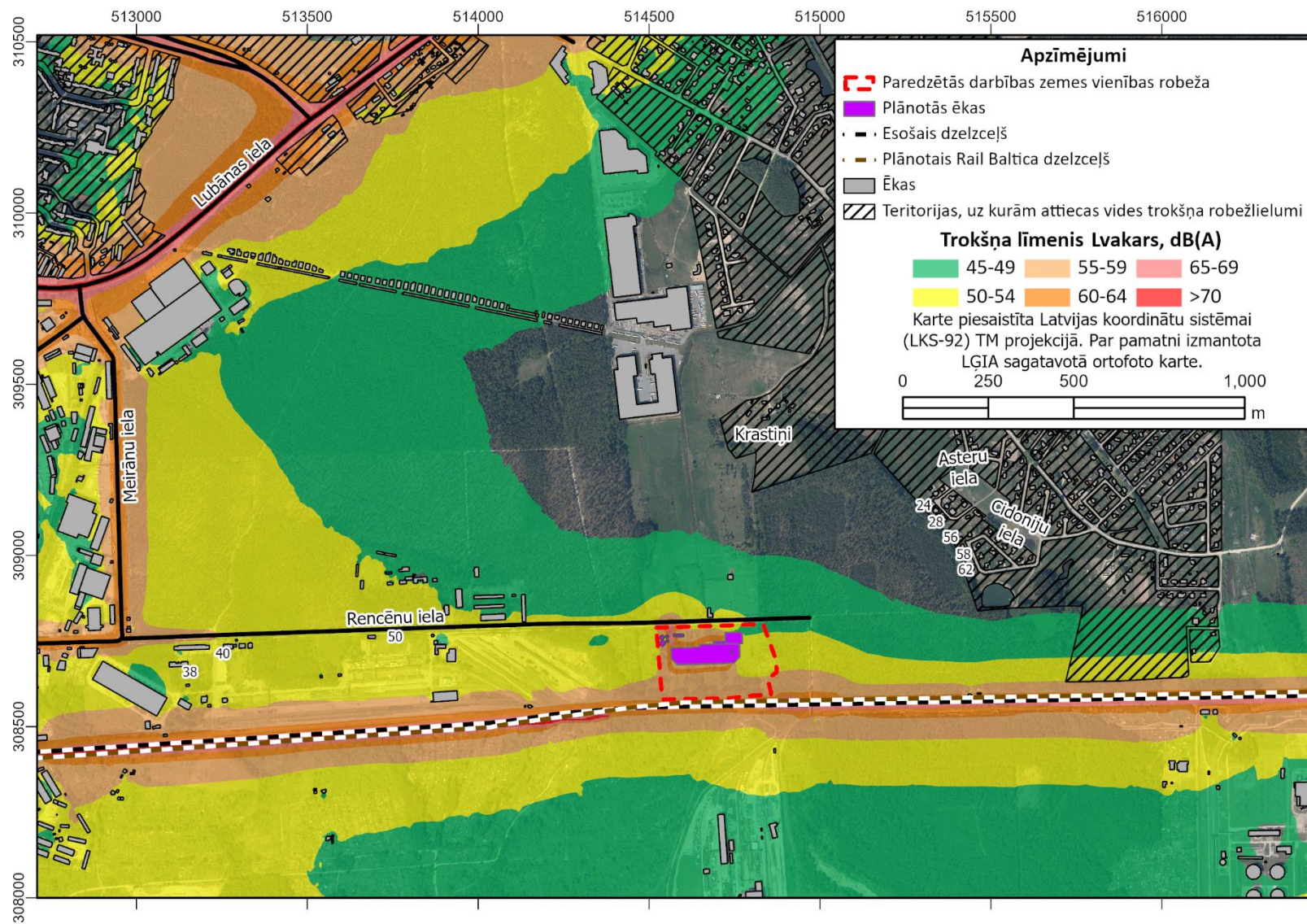
8. attēls. Kopējais sagaidāmais trokšņa līmenis trokšņa rādītājam L_{vakars}
