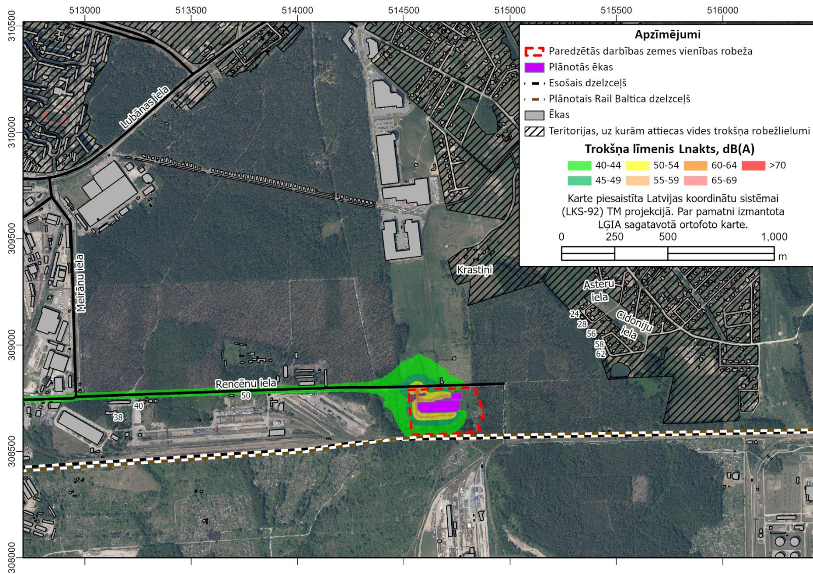
6. attēls. Plānotās darbības radītais trokšņa līmenis trokšņa rādītājam L_{nakts}
