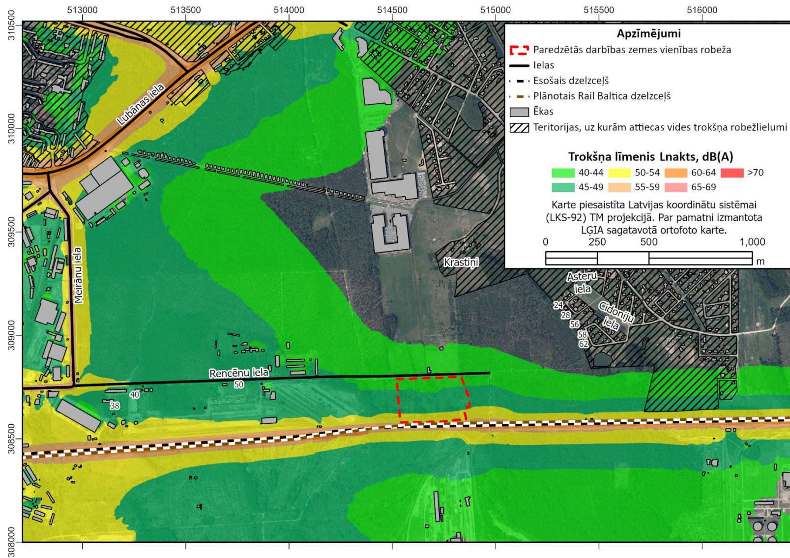
3. attēls. Aprēķinātais fona trokšņa līmenis trokšņa rādītājam L_{nakts}
