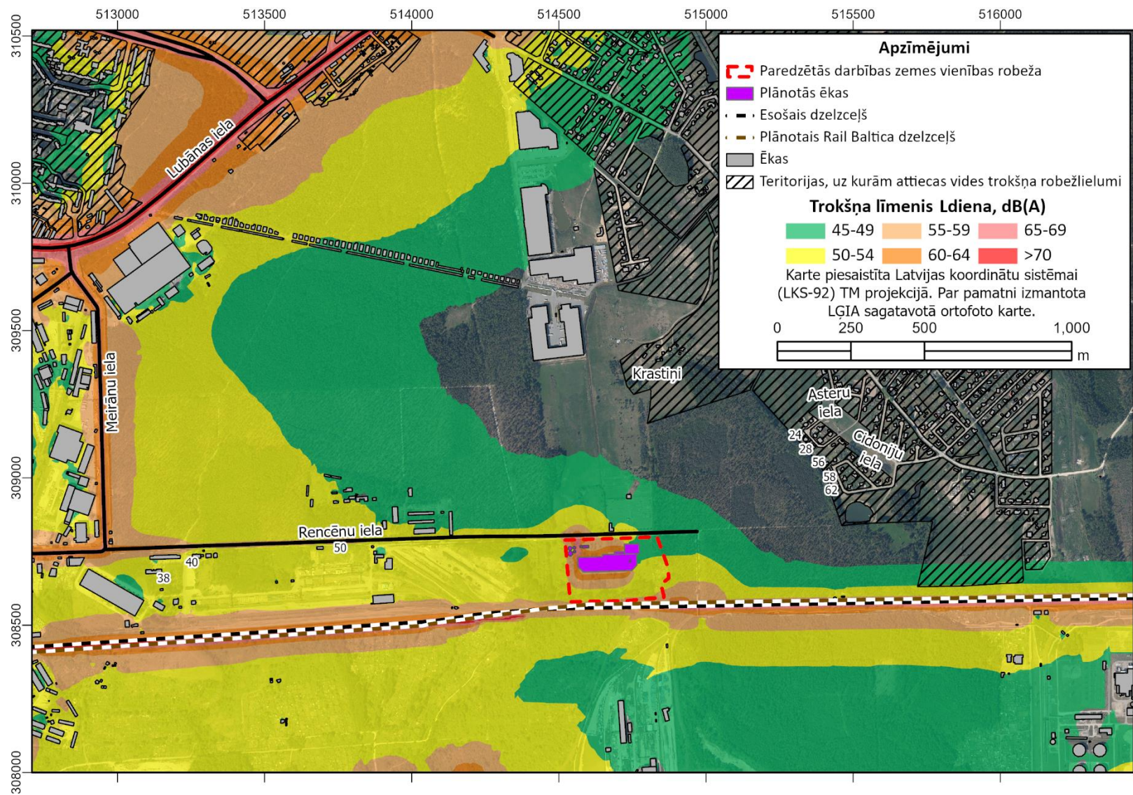
7. attēls. Kopējais sagaidāmais trokšņa līmenis trokšņa rādītājam L_{diena}
