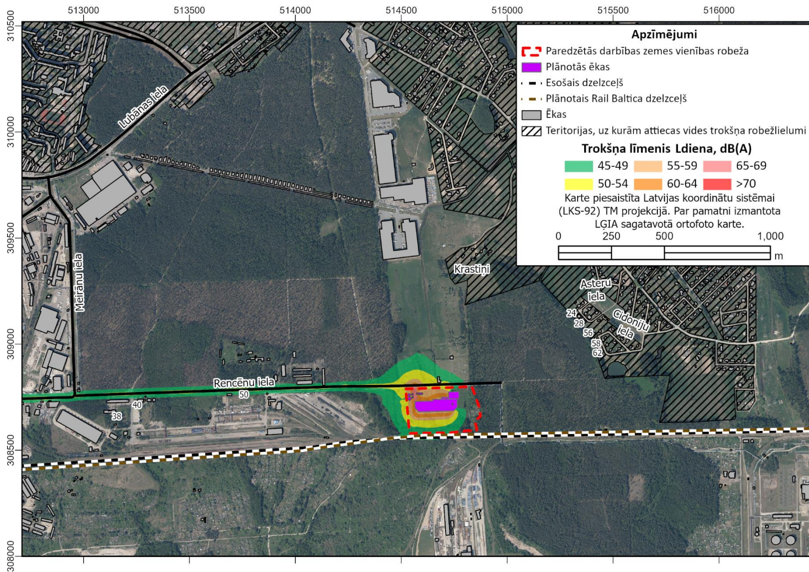
4. attēls. Plānotās darbības radītais trokšņa līmenis trokšņa rādītājam L_{diena}
