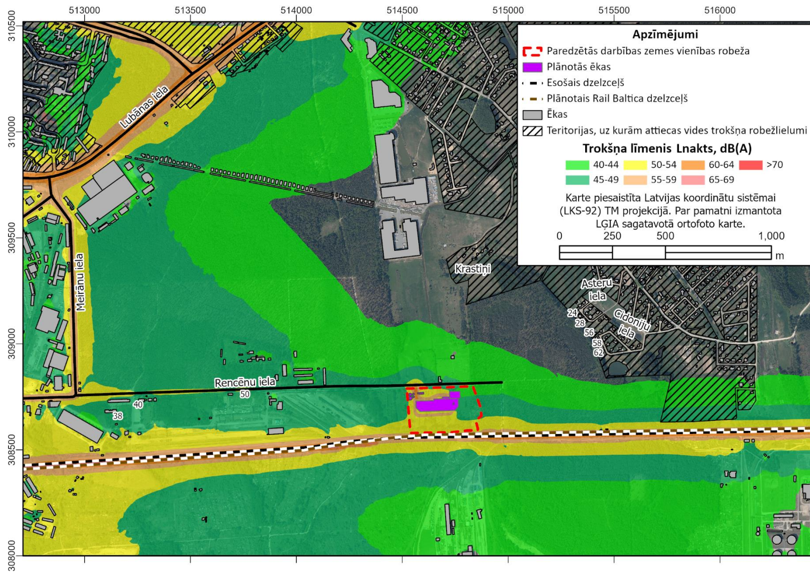
9. attēls. Kopējais sagaidāmais trokšņa līmenis trokšņa rādītājam L_{nakts}
