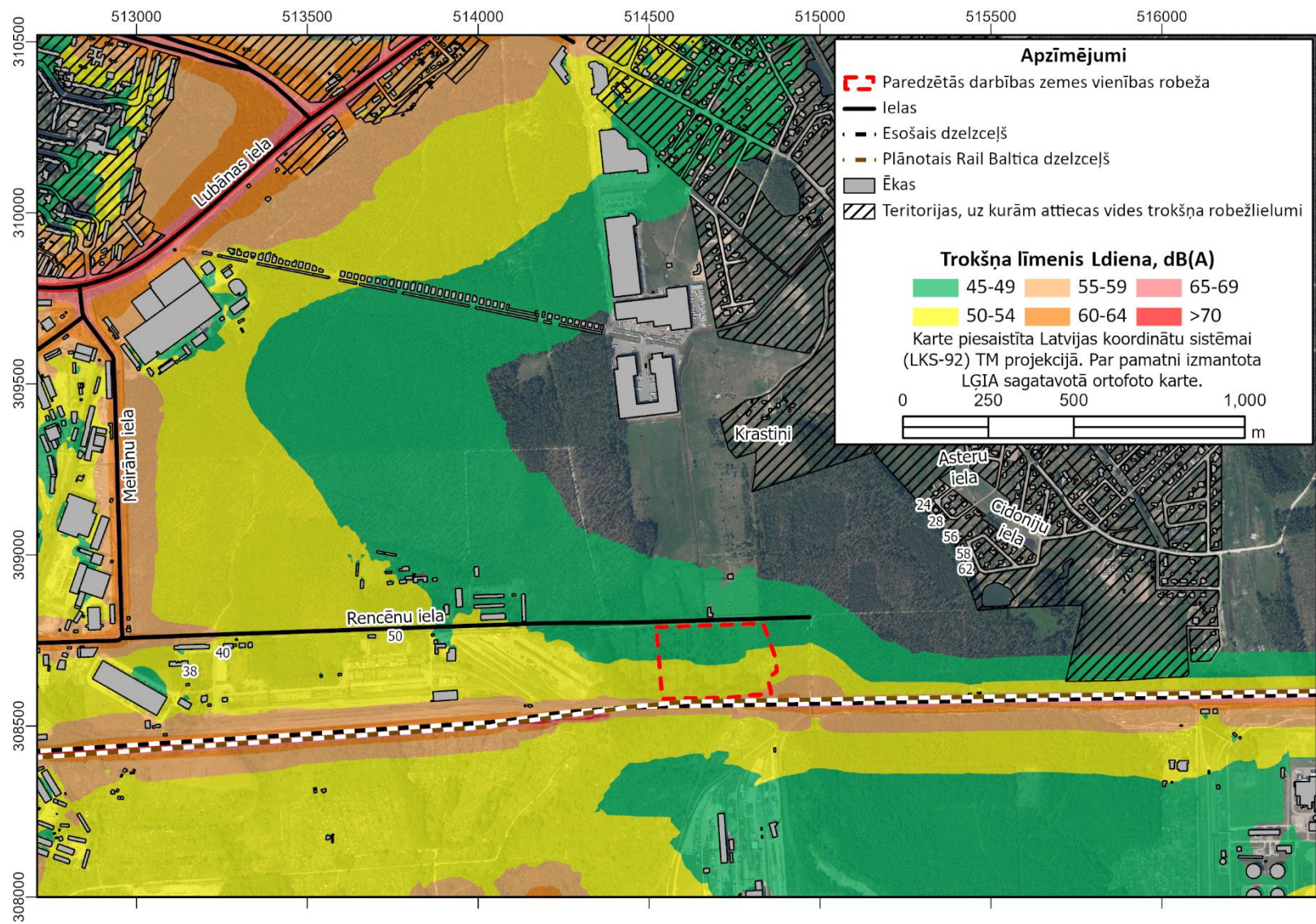
1. attēls. Aprēķinātais fona trokšņa līmenis trokšņa rādītājam L_{diena}
