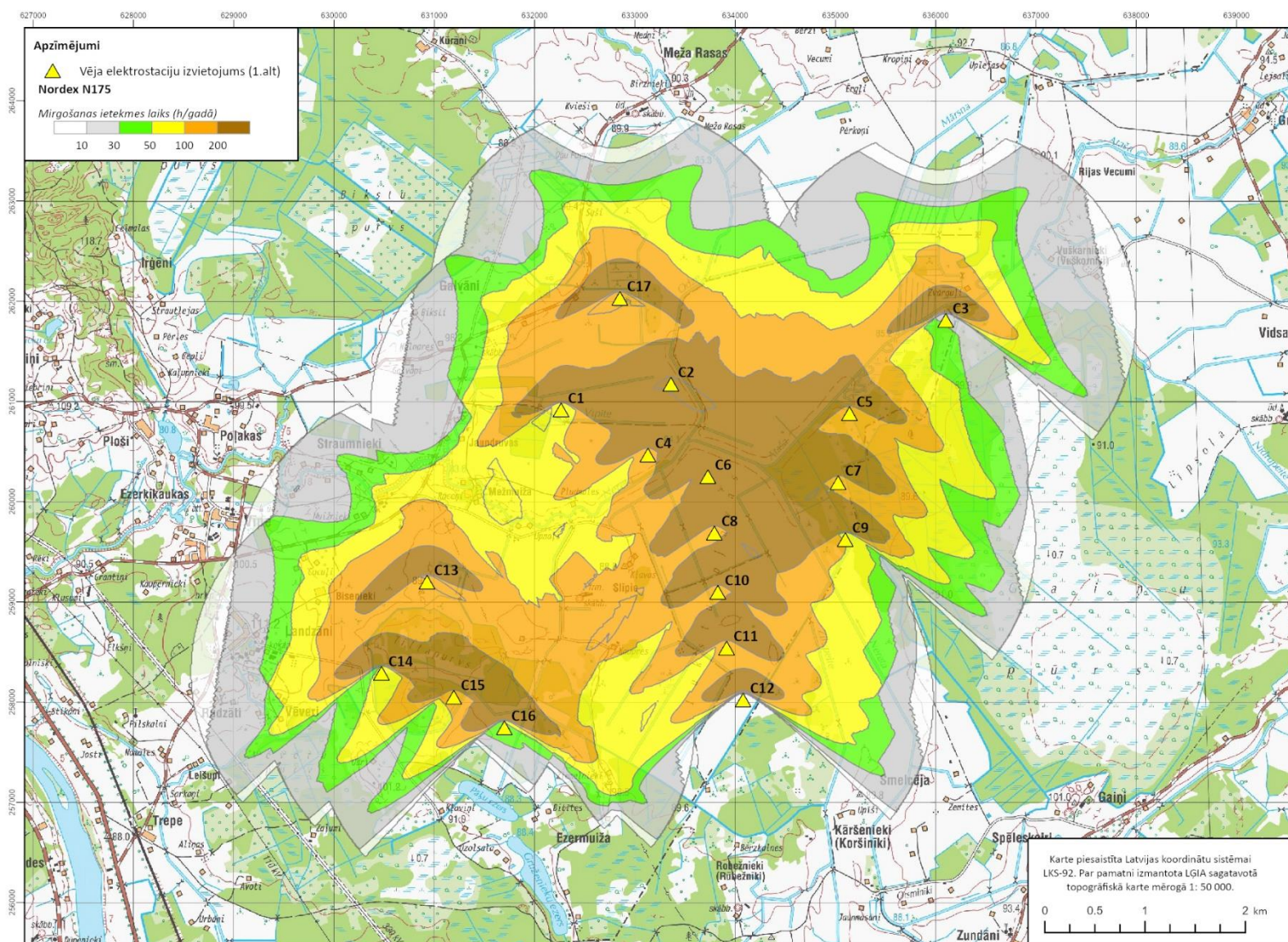
4. attēls. Mirgošanas efekta ietekmes zonas, izbūvējot Nordex N175, izvietojuma C alternatīva
