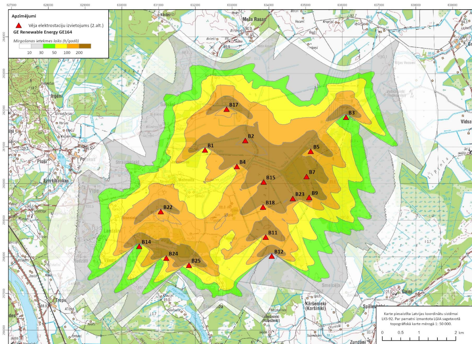
11. attēls. Mirgošanas efekta ietekmes zonas, izbūvējot GE Renewable Energy GE164, izvietojuma B alternatīva
