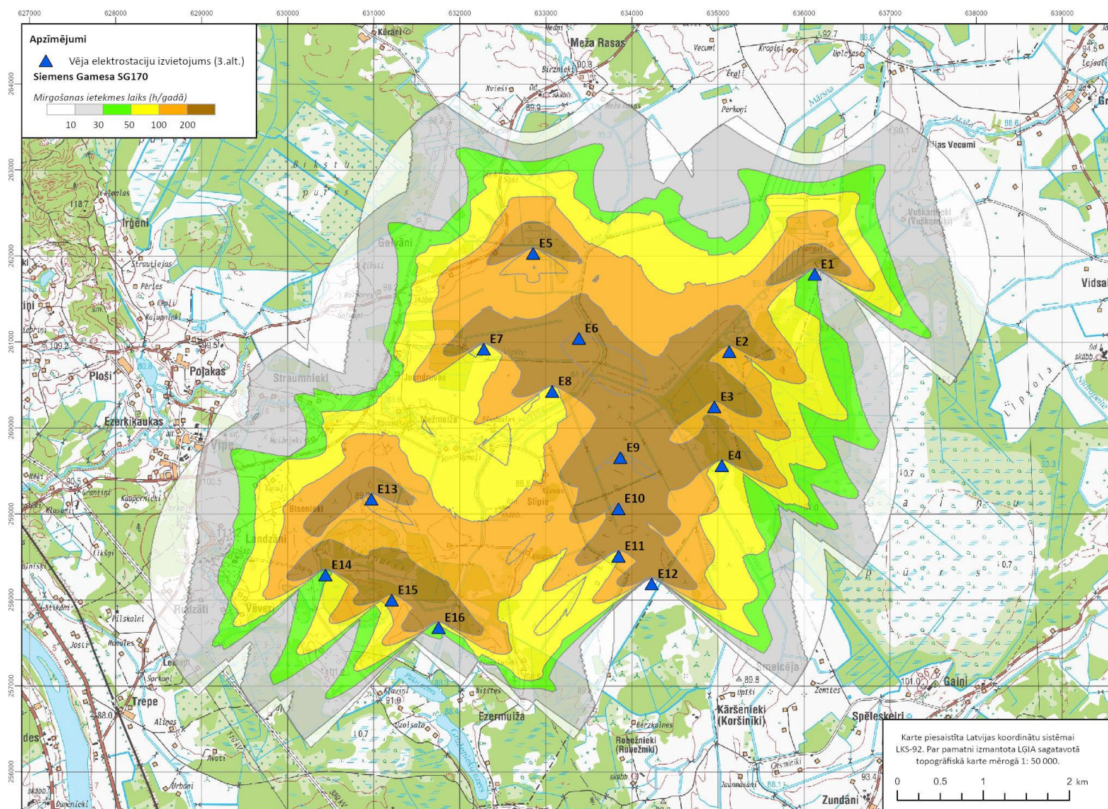
9. attēls. Mirgošanas efekta ietekmes zonas, izbūvējot Siemens Gamesa SG170, izvietojuma E alternatīva
