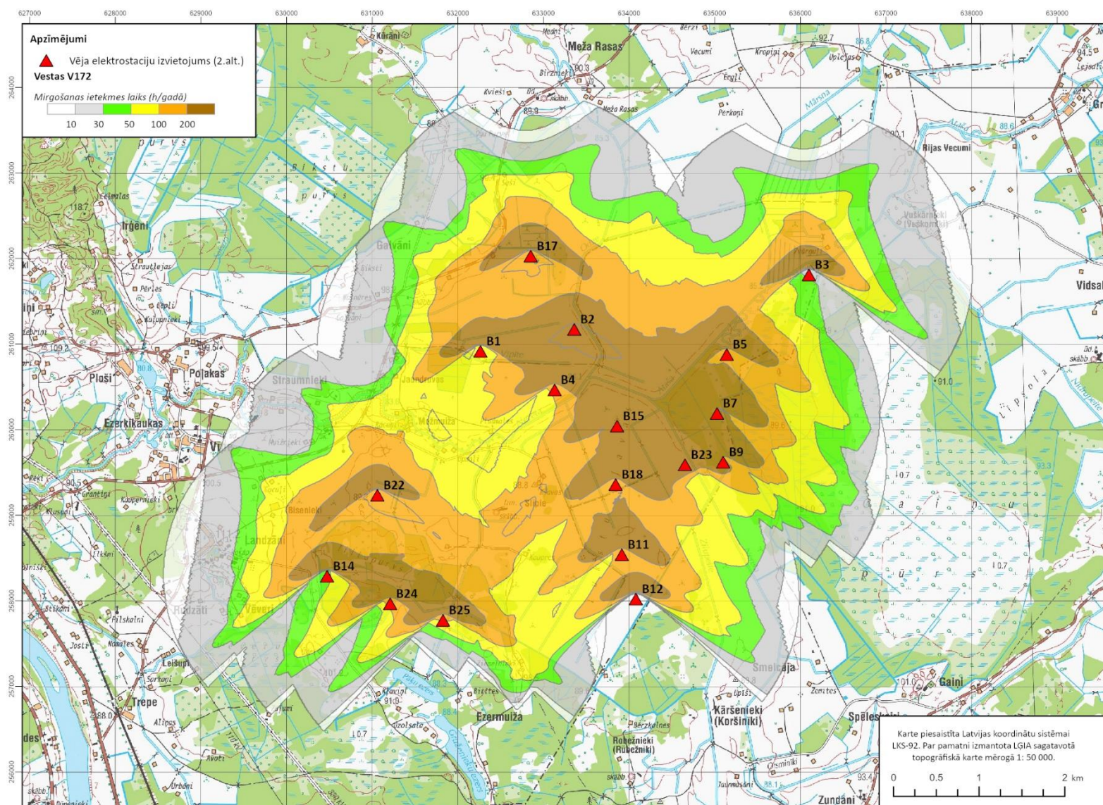
2. attēls. Mirgošanas efekta ietekmes zonas, izbūvējot Vestas V172, izvietojuma B alternatīva
