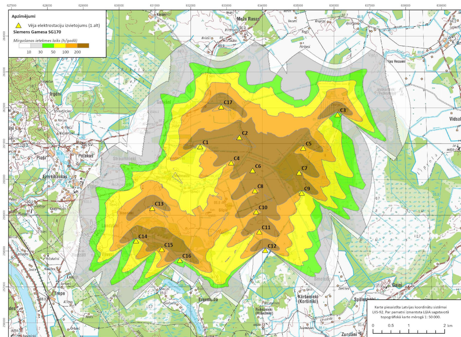
7. attēls. Mirgošanas efekta ietekmes zonas, izbūvējot Siemens Gamesa SG170, izvietojuma C alternatīva
