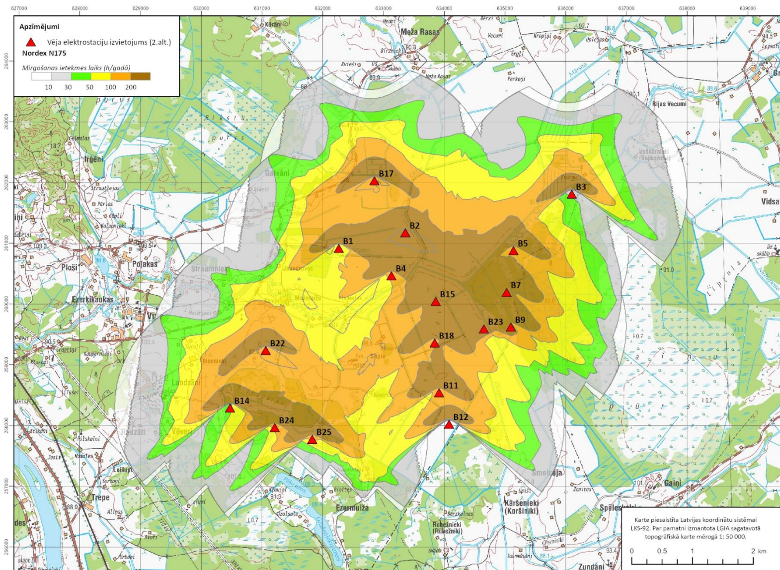
6. attēls. Mirgošanas efekta ietekmes zonas, izbūvējot Nordex N175, izvietojuma E alternatīva
