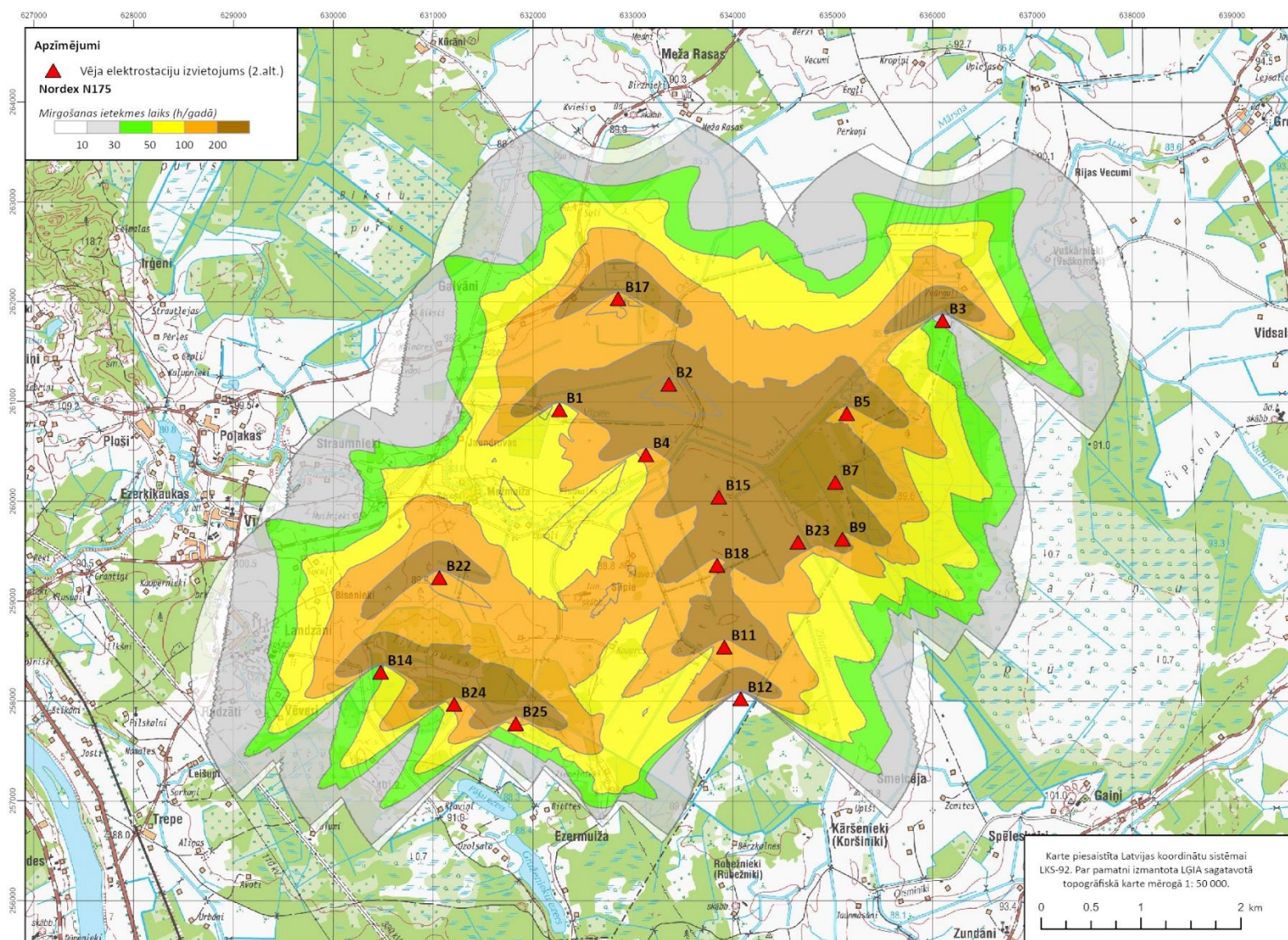
5. attēls. Mirgošanas efekta ietekmes zonas, izbūvējot Nordex N175, izvietojuma B alternatīva
