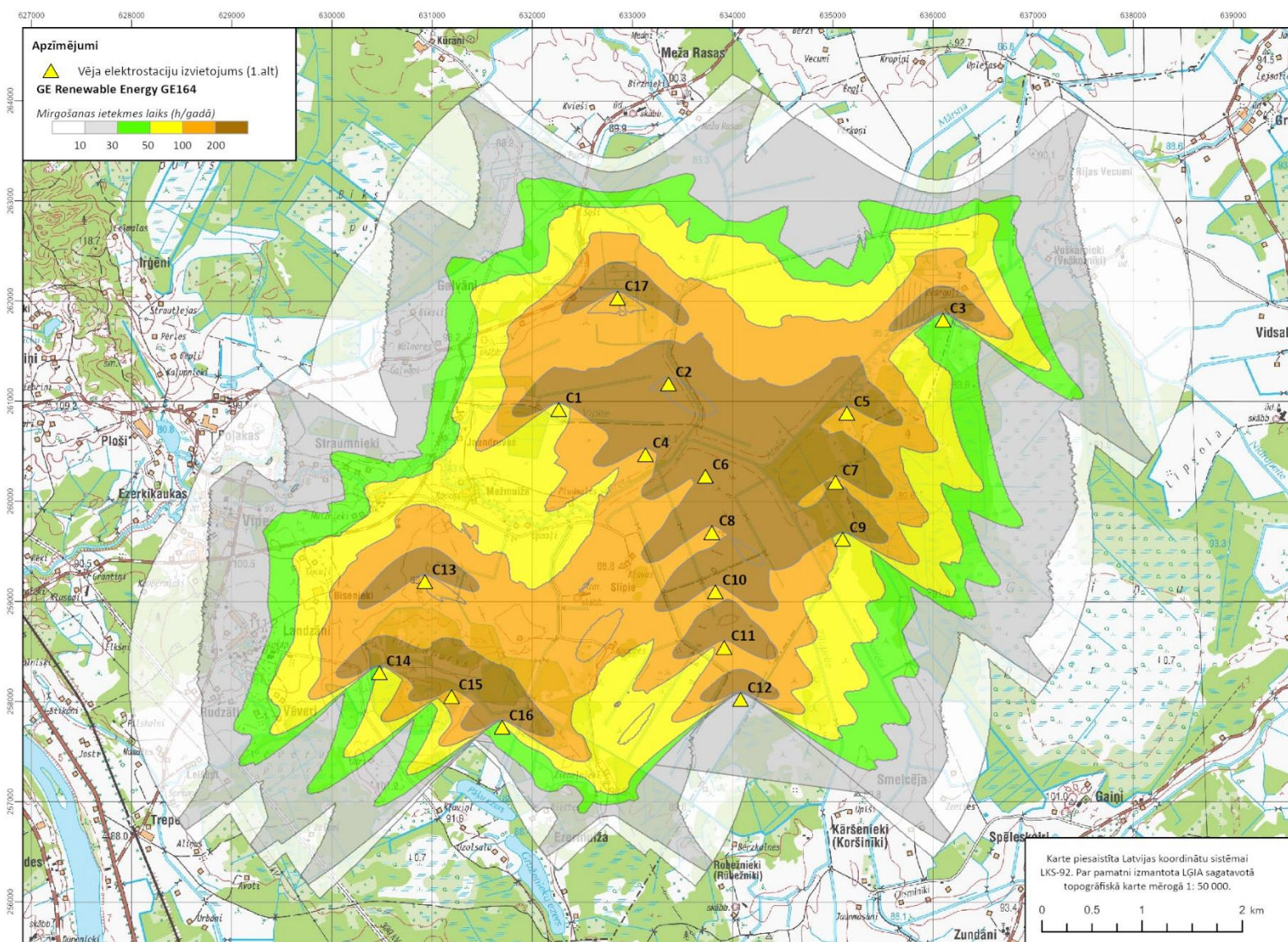
10. attēls. Mirgošanas efekta ietekmes zonas, izbūvējot GE Renewable Energy GE164, izvietojuma C alternatīva
