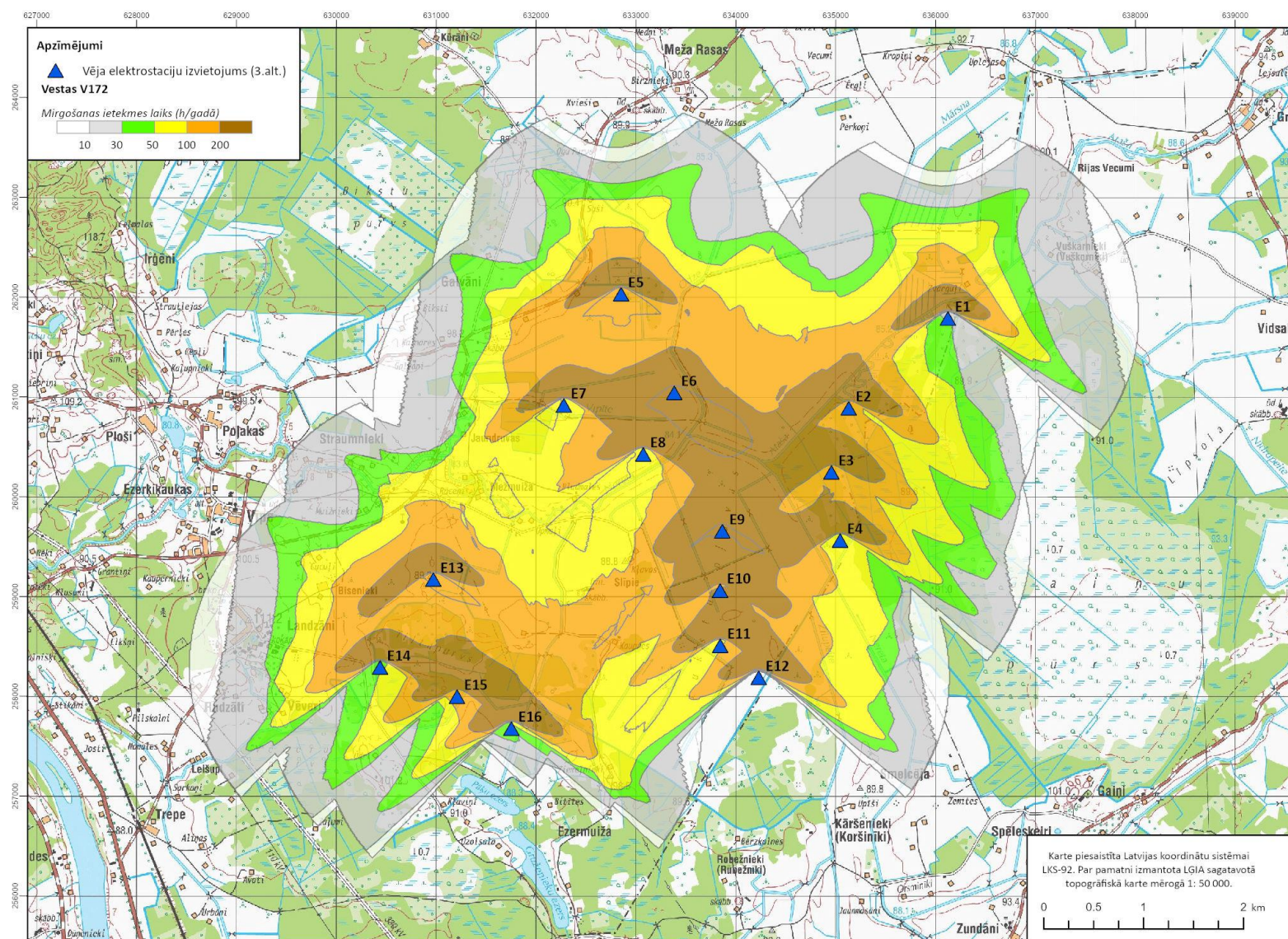
3. attēls. Mirgošanas efekta ietekmes zonas, izbūvējot Vestas V172, izvietojuma E alternatīva
