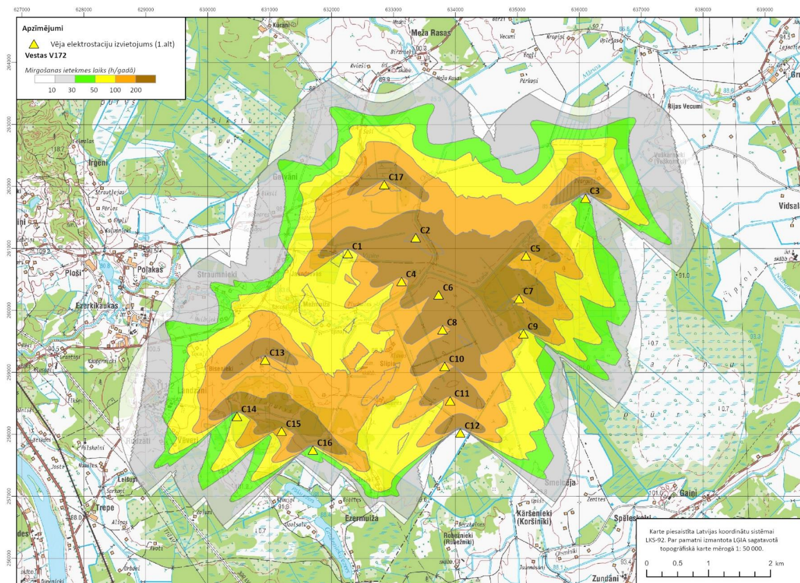
1. attēls. Mirgošanas efekta ietekmes zonas, izbūvējot Vestas V172, izvietojuma C alternatīva
